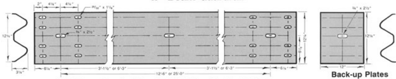
"W"-Beam Guardrail Per AASHTO Specification M-180
